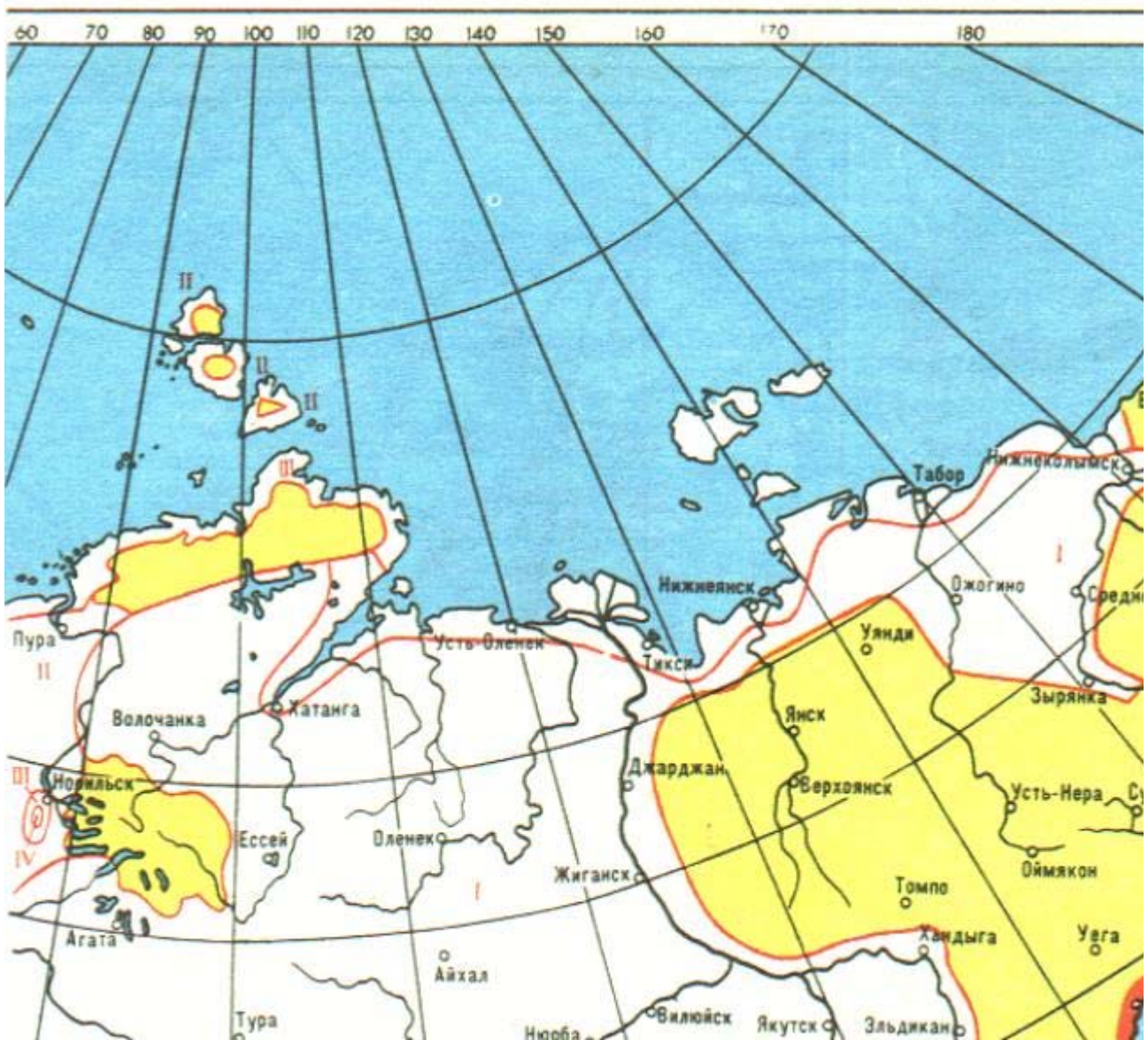
Рис. 2.5.7. Карта районирования территории по толщине стенки гололеда. Лист 3
