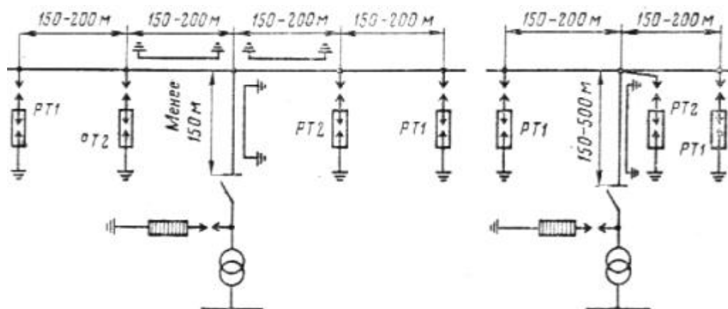
Рис. 4.2.16. Схемы защиты от грозвых перенапряжении подстанций, присоединенных к ВЛ ответвлениями длиной до 150 и более 150 м
