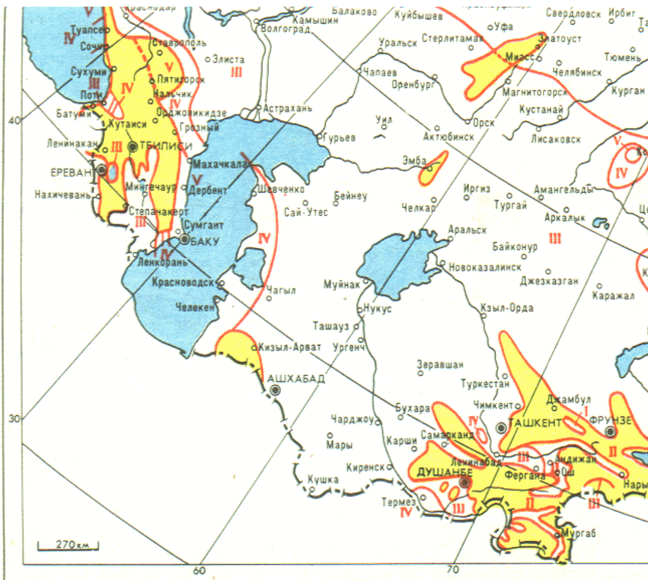
Рис. 2.5.2. Карта районирования территории по скоростным напорам ветра. Лист 2
