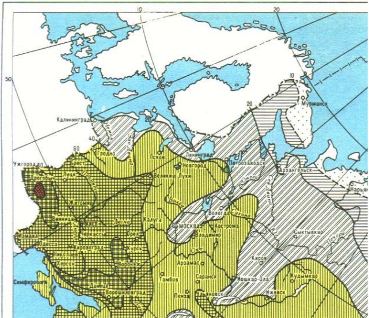
Рис. 2.5.13. Карта среднегодовой продолжительности гроз. Лист 1
