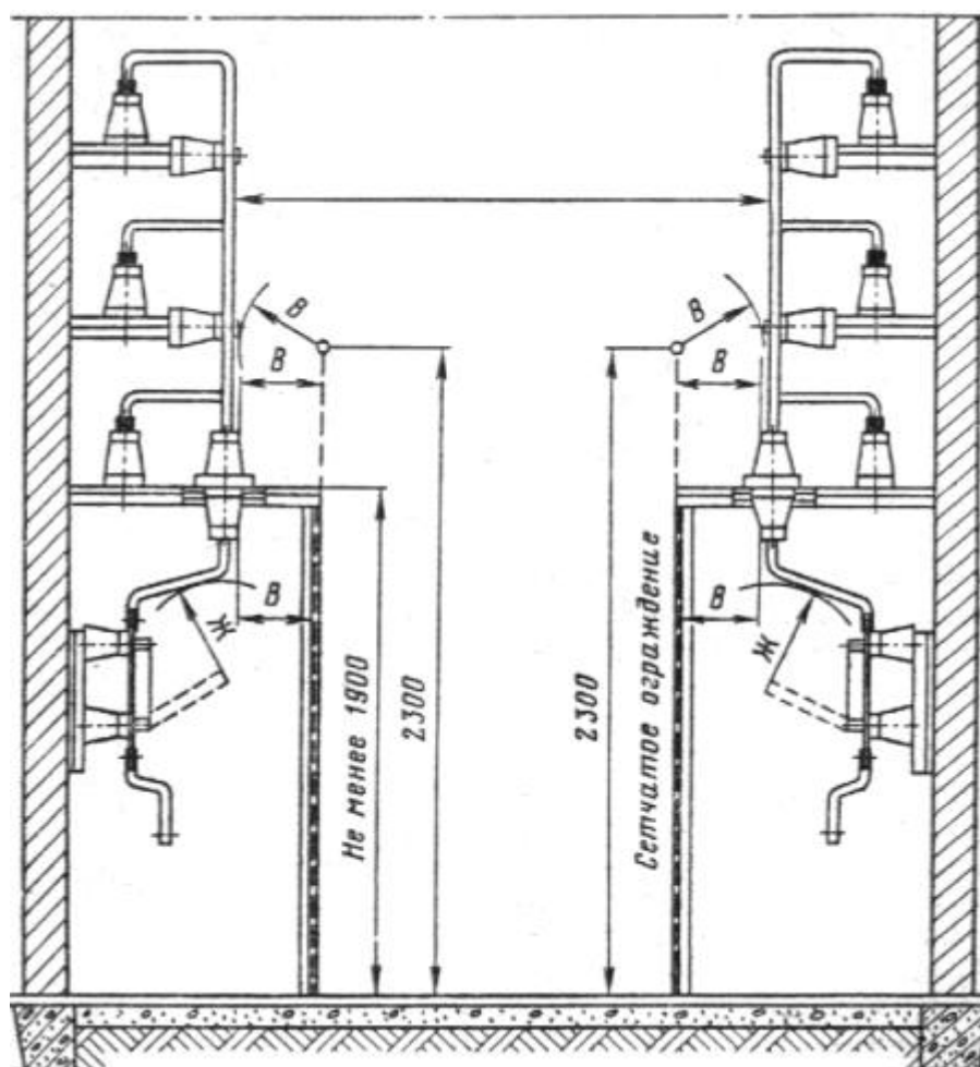
Рис. 4.2.14. Наименьшие расстояния от неизолированных токоведущих частей в ЗРУ до сетчатых ограждений и между неограженными неизолированными токоведущими частями разных цепей (по табл. 4.2.5)
