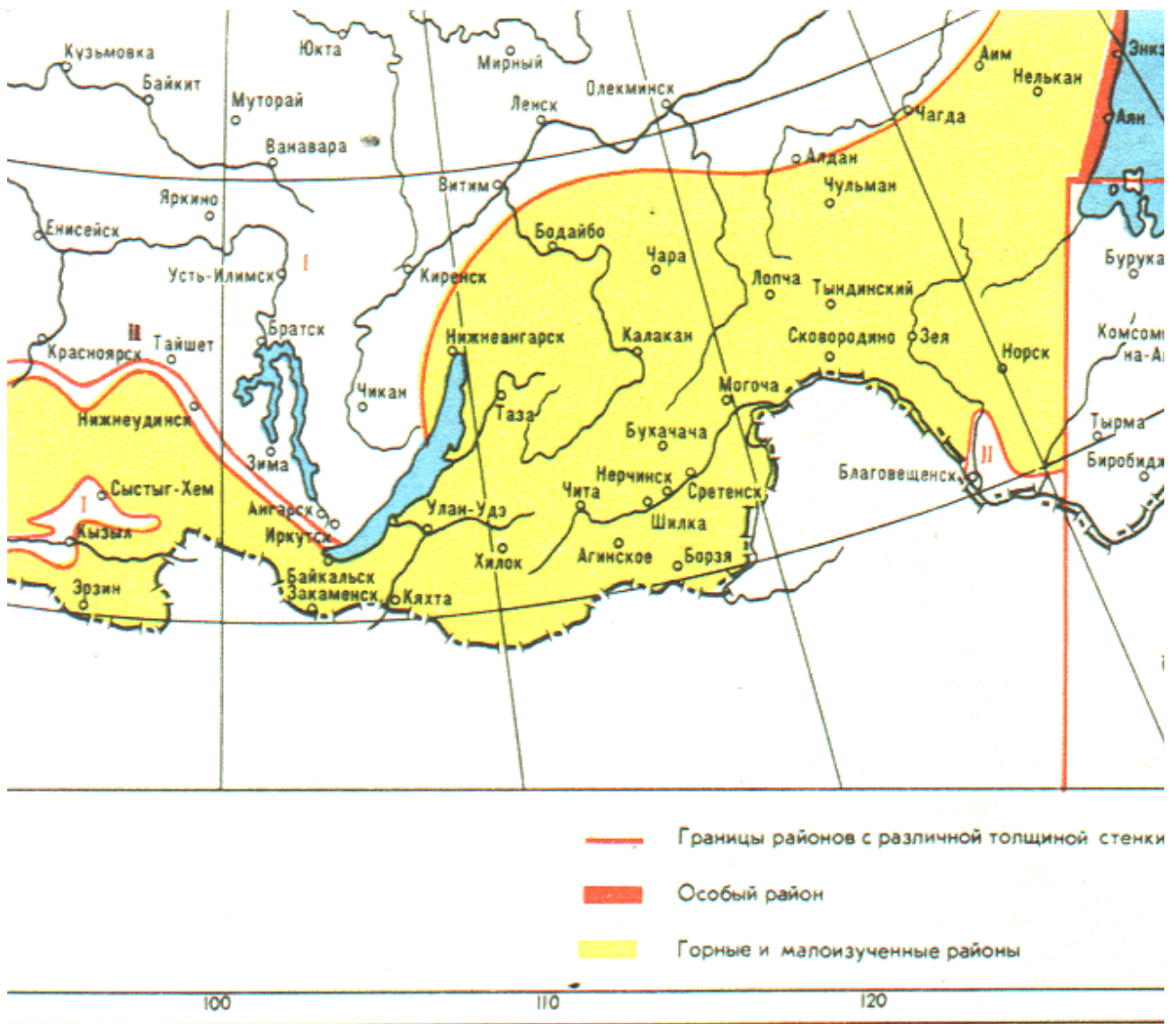
Рис. 2.5.8. Карта районирования территории по толщине стенки гололеда. Лист 4
