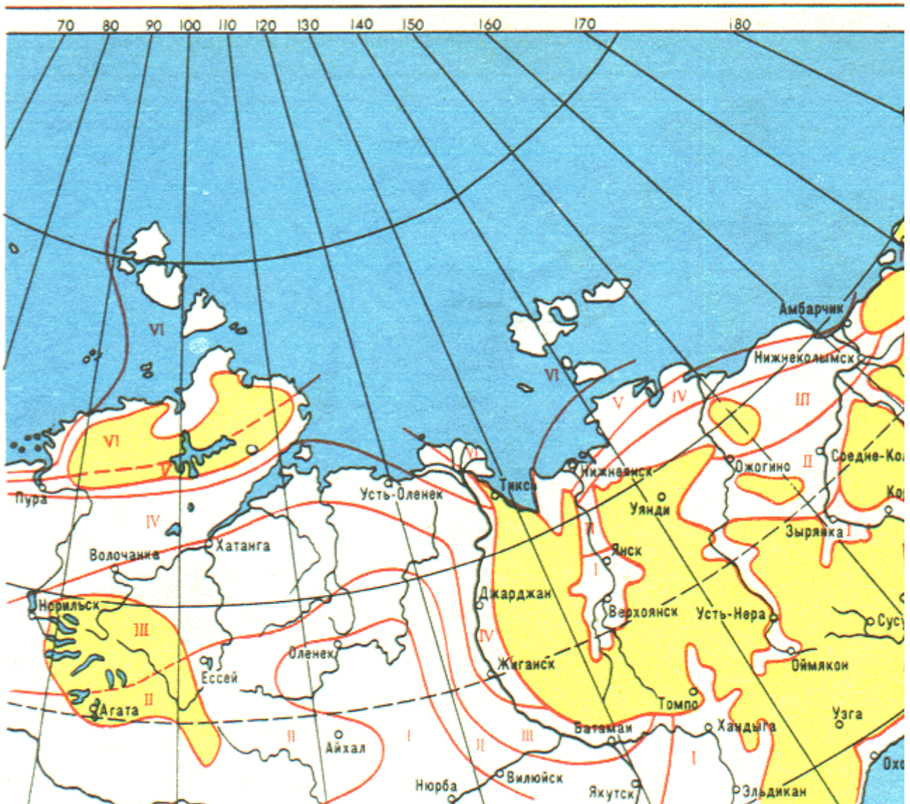
Рис. 2.5.3. Карта районирования территории по скоростным напорам ветра. Лист 3
