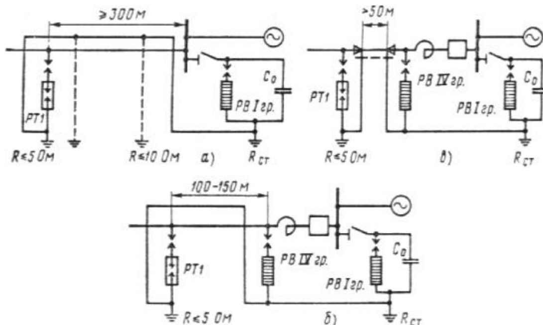
Рис. 4.2.18. Схемы защиты вращающихся машин от грозовых перенапряжений
