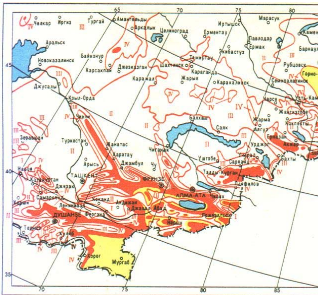
Рис. 2.5.9. Карта районирования территории по толщине стенки гололеда. Лист 5
