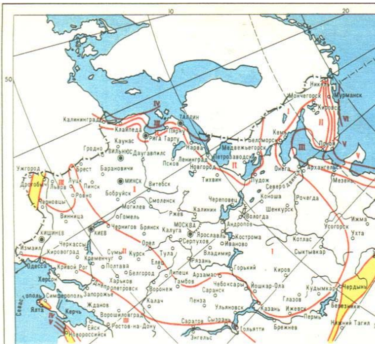
Рис. 2.5.1. Карта районирования территории по скоростным напорам ветра.
