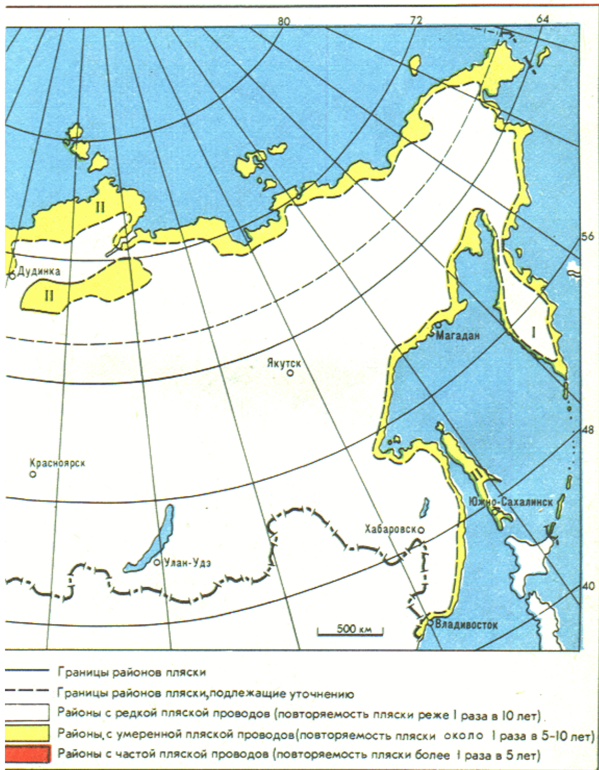
Рис. 2.5.12. Карта районирования территории по пляске проводов.
