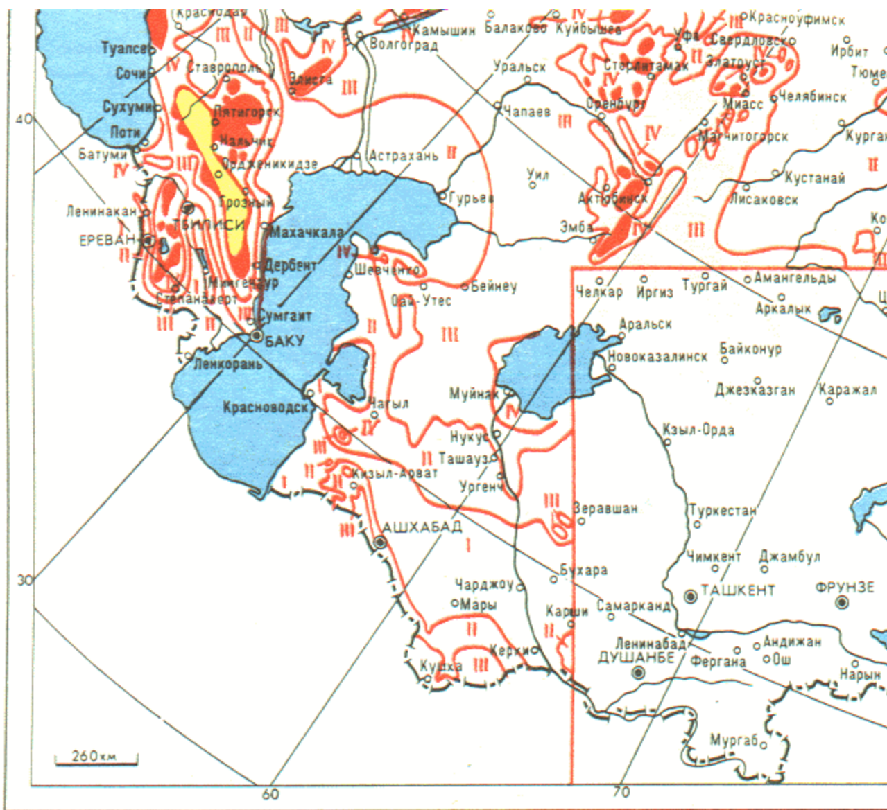
Рис. 2.5.6. Карта районирования территории по толщине стенки гололеда. Лист 2
